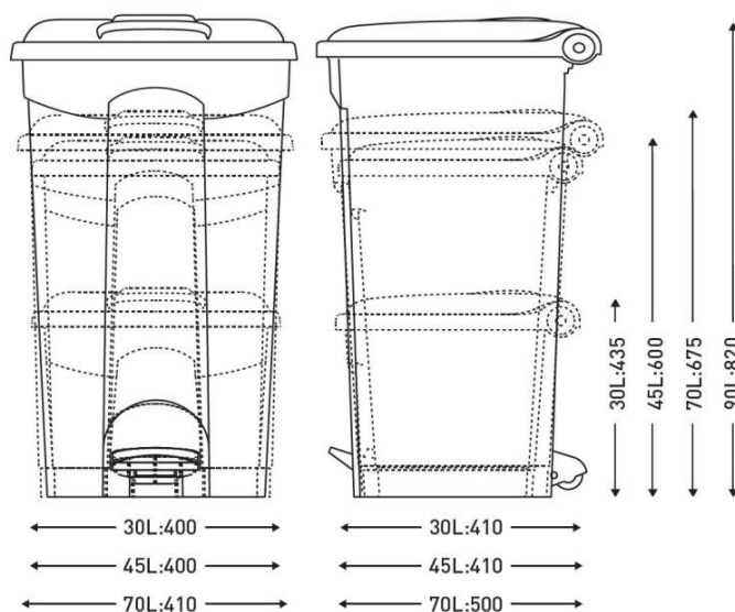
DIBUJO TÉCNICO
