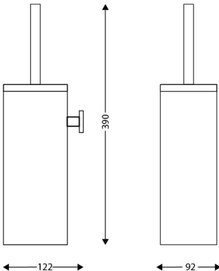
TECHNISCHE ZEICHNUNG
