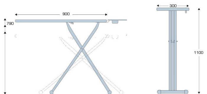
TECHNISCHE ZEICHNUNG
