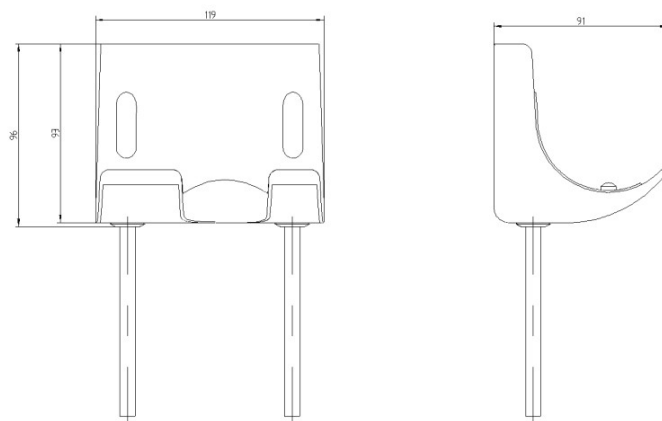
TECHNISCHE ZEICHNUNG
