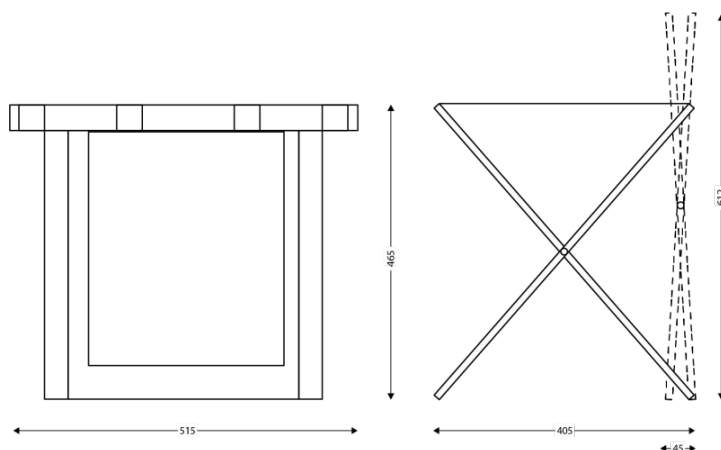
DIBUJO TÉCNICO
