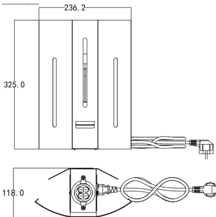
TECHNISCHE ZEICHNUNG
