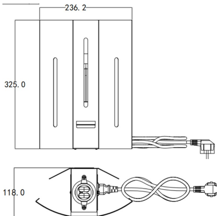
TECHNISCHE ZEICHNUNG
