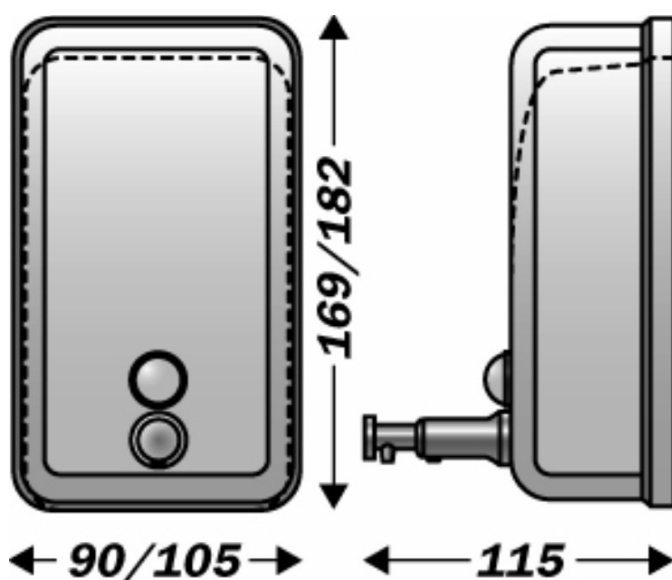
DESSIN TECHNIQUE
