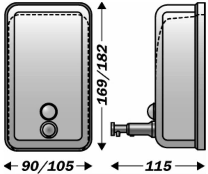
DESSIN TECHNIQUE
