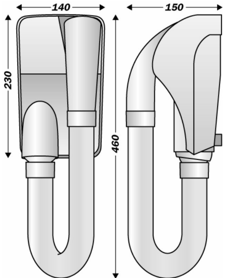
TECHNISCHE ZEICHNUNG
