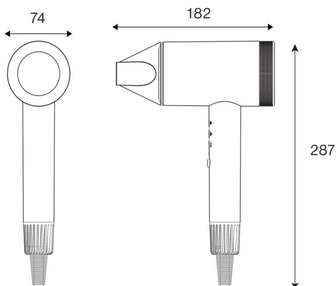
DIBUJO TÉCNICO
