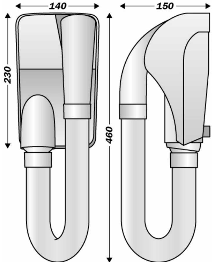
DESSIN TECHNIQUE
