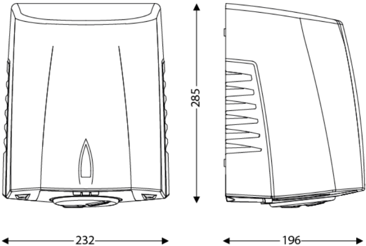
DIBUJO TÉCNICO
