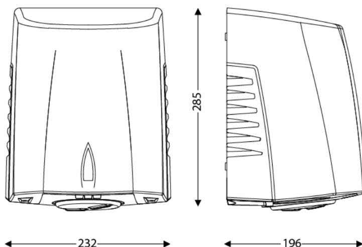
DIBUJO TÉCNICO
