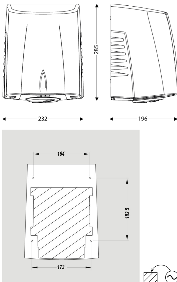
TECHNISCHE ZEICHNUNG
