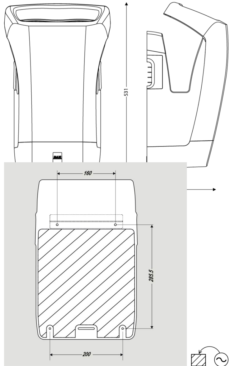
DIBUJO TÉCNICO
